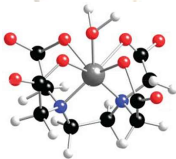
[MgEDTA(H_2O)]^{2-} (2 分)
